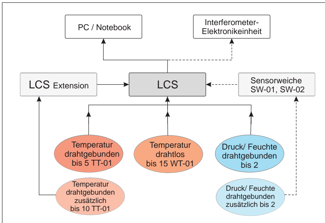
Klimamessstation LCS-01 mit Funk (Artikel-Nr. A032123) Klimamessstation LCS-02 ohne Funk (Artikel-Nr. A032124)
